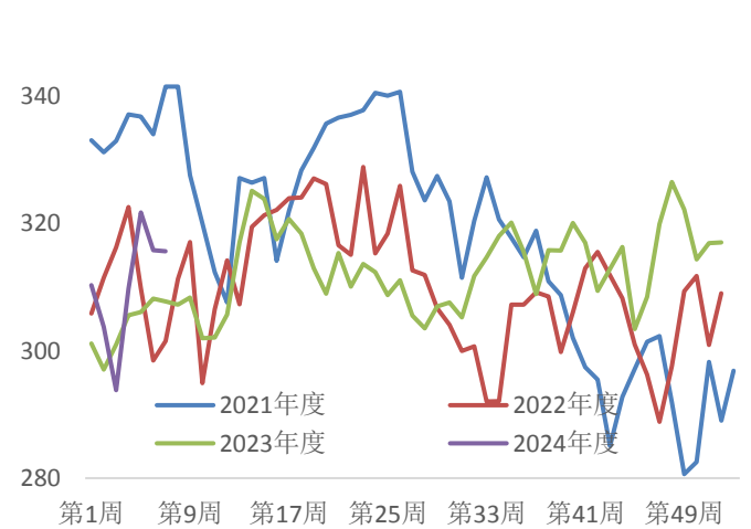
图 16: 热卷周度产量 单位: 万吨
