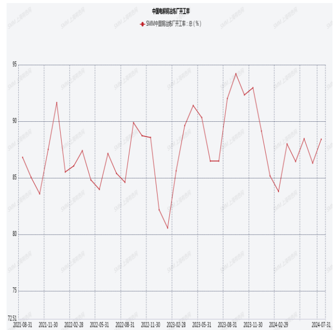
图 20 中国电解铜冶炼企业开工率
